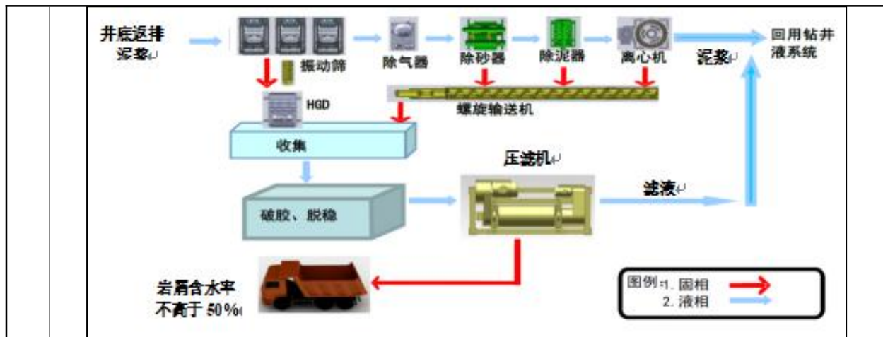
图2-6 泥浆循环系统工艺流程简图
