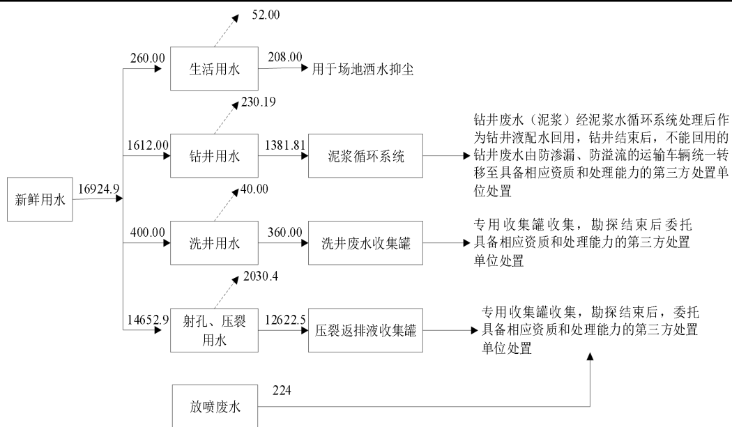
图2-5 项目水平衡图（单位：m³/施工期）
