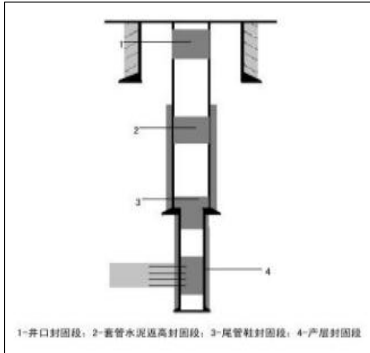
图 2-4 永久封井剖面示意图
