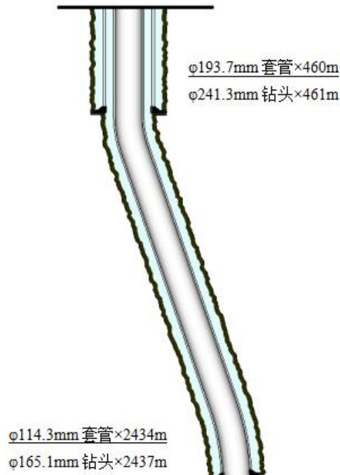
佳南403井身结构示意图 图2-2 井身结构示意图
