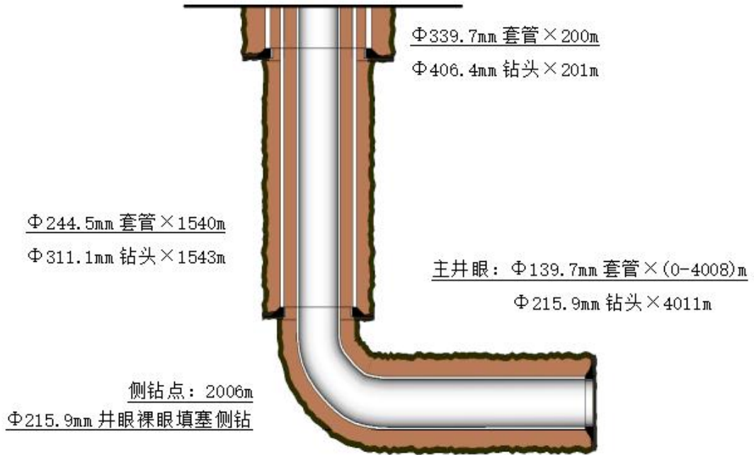
佳南 303H 井身结构示意图
