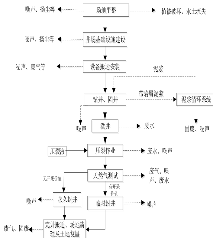
图2-7 项目主要工艺流程及产污环节
