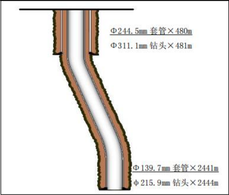
图 2-1 井身结构示意图
