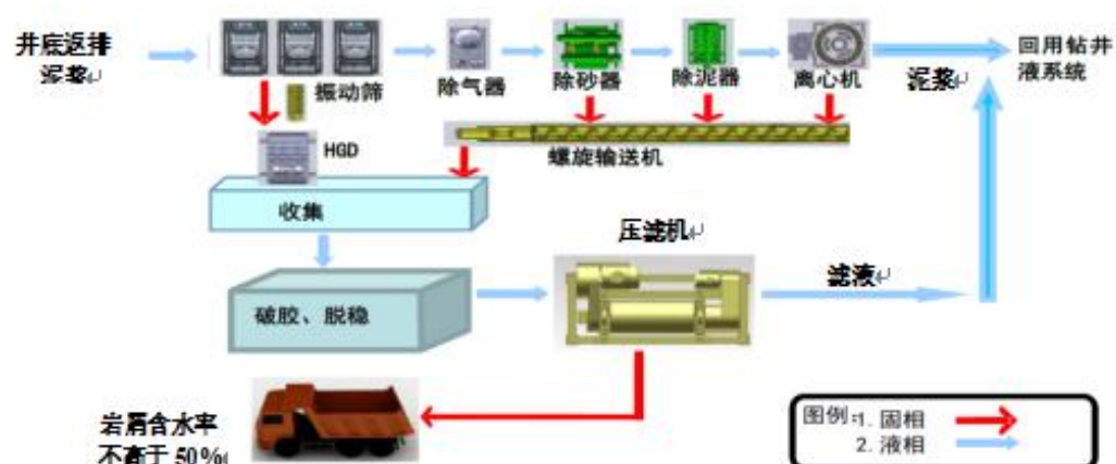
图2-5 泥浆循环系统工艺流程简图
