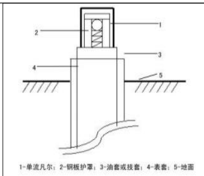
图2-2 临时封井示意图
