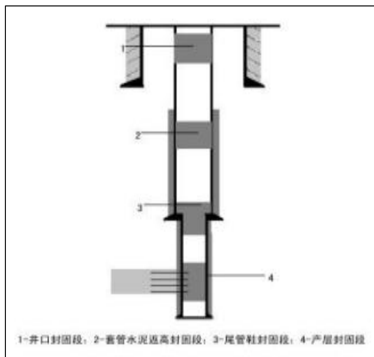
图 2-3 永久封井剖面示意图
